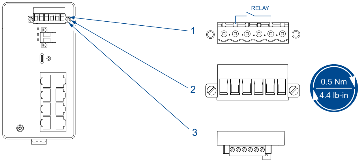
Abb. 6: (1) Anschluss am Gerät, (2) Klemmblock montiert am Gerät (Vorderansicht), Anzugsdrehmoment, (3) Klemmblock montiert am Gerät (Ansicht von oben).
