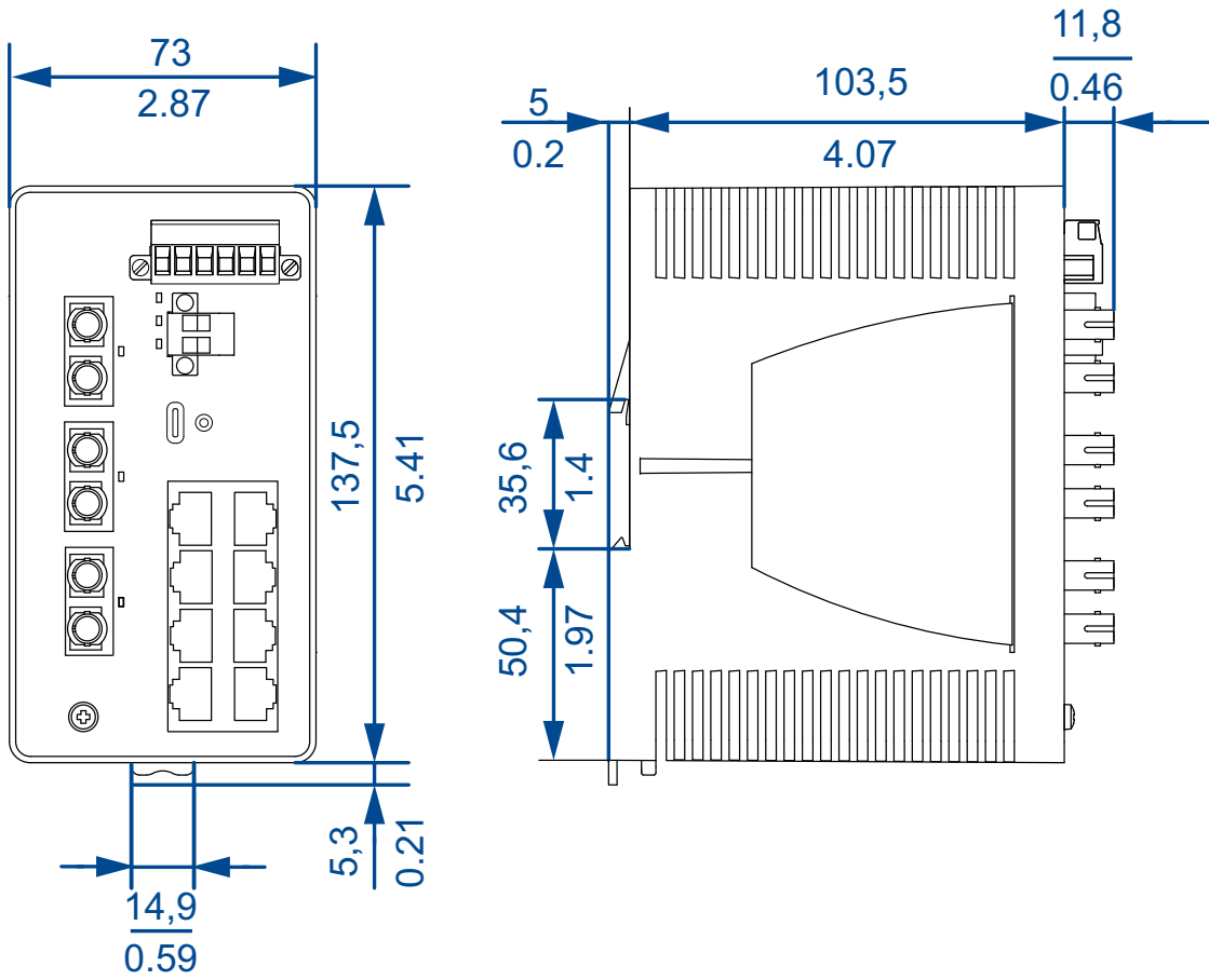
Abb. 25: Gerätevarianten im mittleren Kunststoffgehäuse
