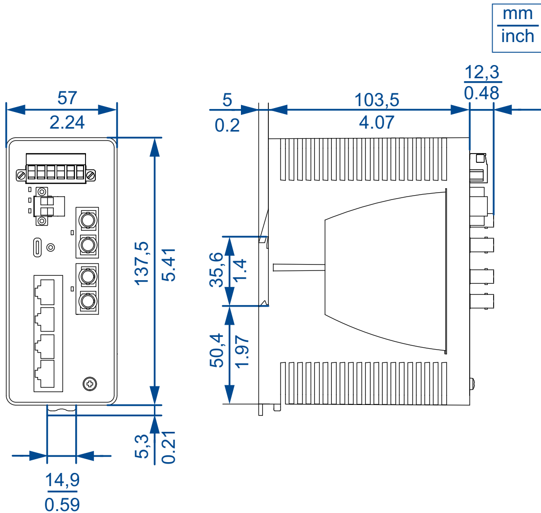
Abb. 24: Gerätevarianten im schmalen Kunststoffgehäuse
