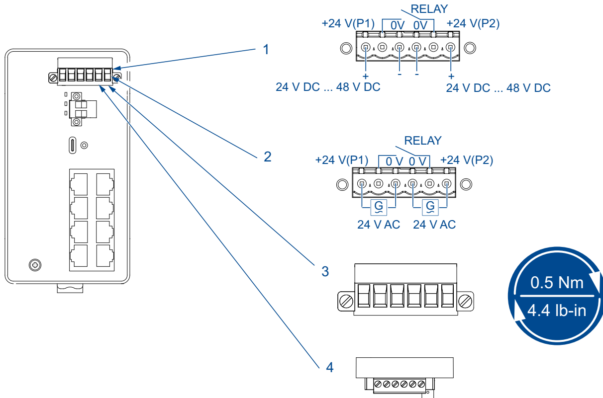
Abb. 15: (1) Gleichspannung-Anschluss am Gerät, (2) Wechselspannung-Anschluss am Gerät, (3) Klemmblock montiert am Gerät (Vorderansicht), Anzugsdrehmoment, (4) Klemmblock montiert am Gerät (Ansicht von oben).
