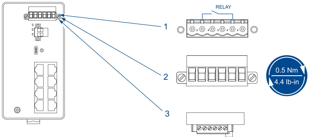
Abb. 18: (1) Anschluss am Gerät, (2) Klemmblock montiert am Gerät (Vorderansicht), Anzugsdrehmoment, (3) Klemmblock montiert am Gerät (Ansicht von oben).
