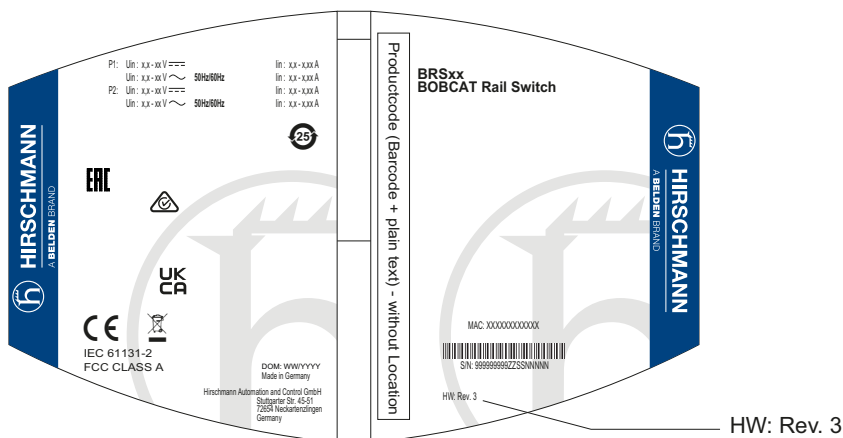
Abb. 10: Revision-Kennzeichnung auf dem Seitenlabel
