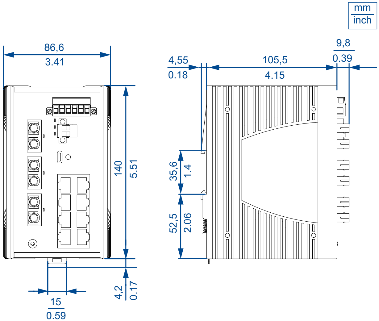
Abb. 28: Gerätevarianten im mittleren Metallgehäuse
