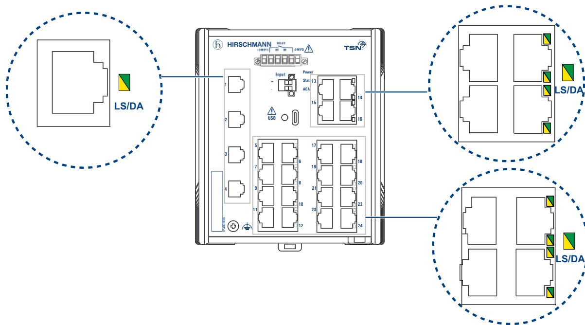
Abb. 5: LED-Anzeigeelemente bei einer High-Port-Gerätevariante mit SFP-Schächten und 20 x RJ45-Buchsen
