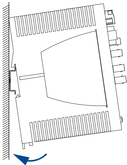
Abb. 11: Montage auf die Hutschiene
