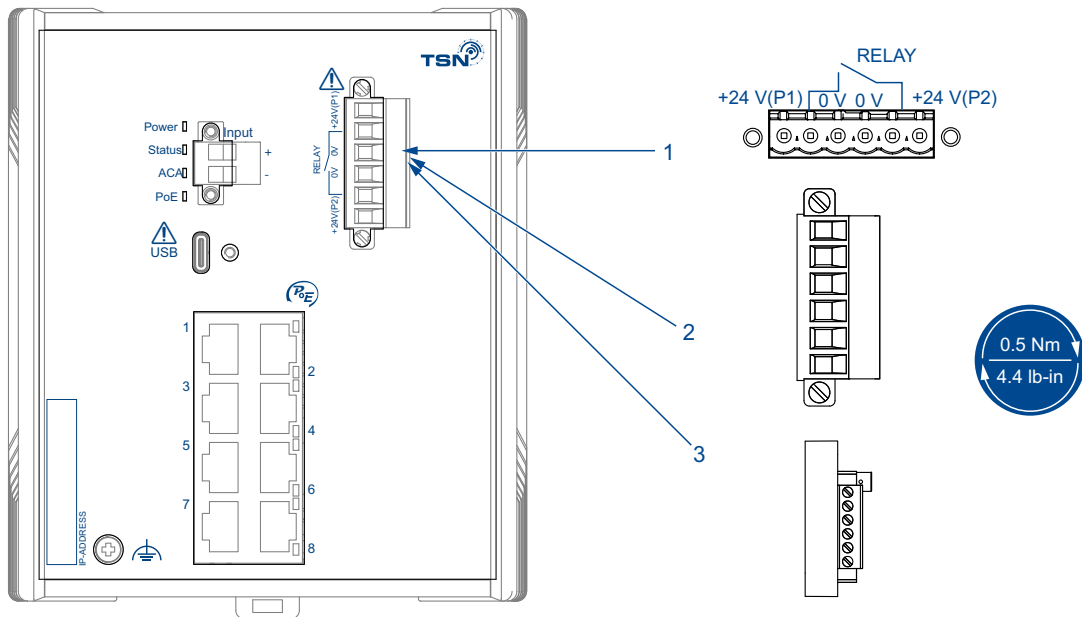
Abb. 16: (1) Gleichspannung-Anschluss am Gerät, (2) Klemmblock montiert am Gerät (Vorderansicht), Anzugsdrehmoment, (3) Klemmblock montiert am Gerät (Ansicht von oben).
