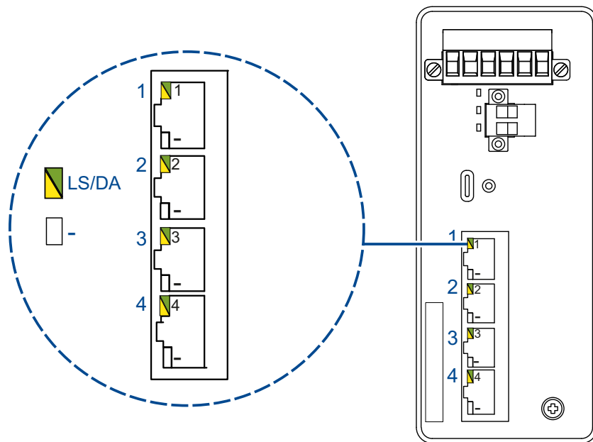
Abb. 2: LED-Anzeigeelemente bei Gerätevarianten mit 4 × RJ45-Buchsen
