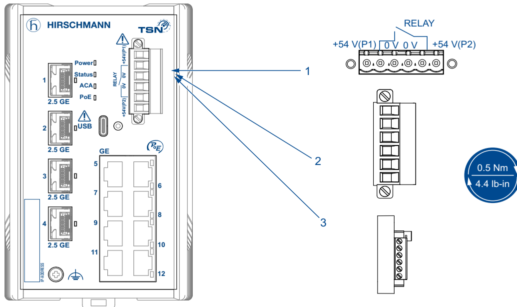
Abb. 17: (1) Gleichspannung-Anschluss am Gerät, (2) Klemmblock montiert am Gerät (Vorderansicht), Anzugsdrehmoment, (3) Klemmblock montiert am Gerät (Ansicht von oben).
