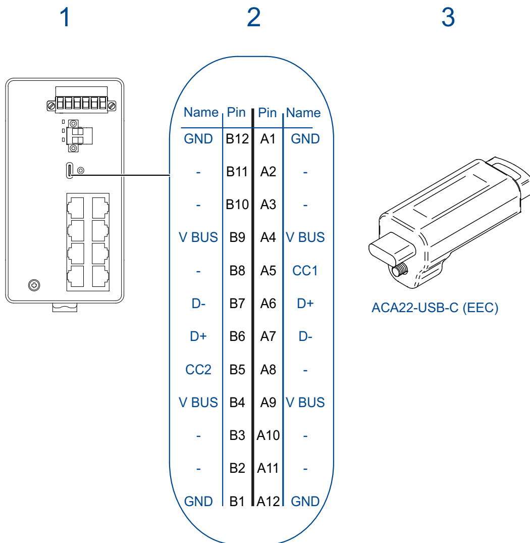
Abb. 7: (1) Position der USB-C-Schnittstelle am Gerät, (2) Pinbelegung der USB-C-Schnittstelle, (3) Ansicht des ACA22-USB-C (EEC).
