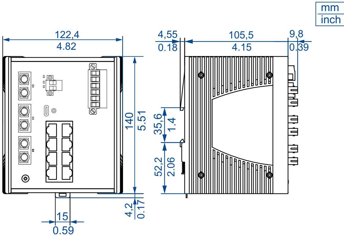
Abb. 29: Gerätevarianten im breiten Metallgehäuse
