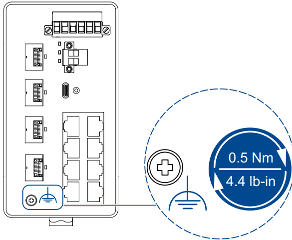
Abb. 12: Position des Erdungsanschlusses am Gerät, Anzugsdrehmoment.
