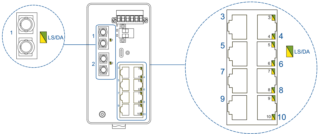
Abb. 3: LED-Anzeigeelemente bei Gerätevarianten mit DSC-, DST- und 8 x RJ45-Buchsen
