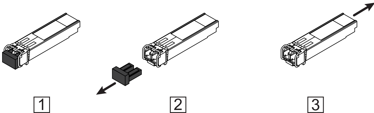
Abb. 13: SFP-Transceiver montieren: Montagereihenfolge
