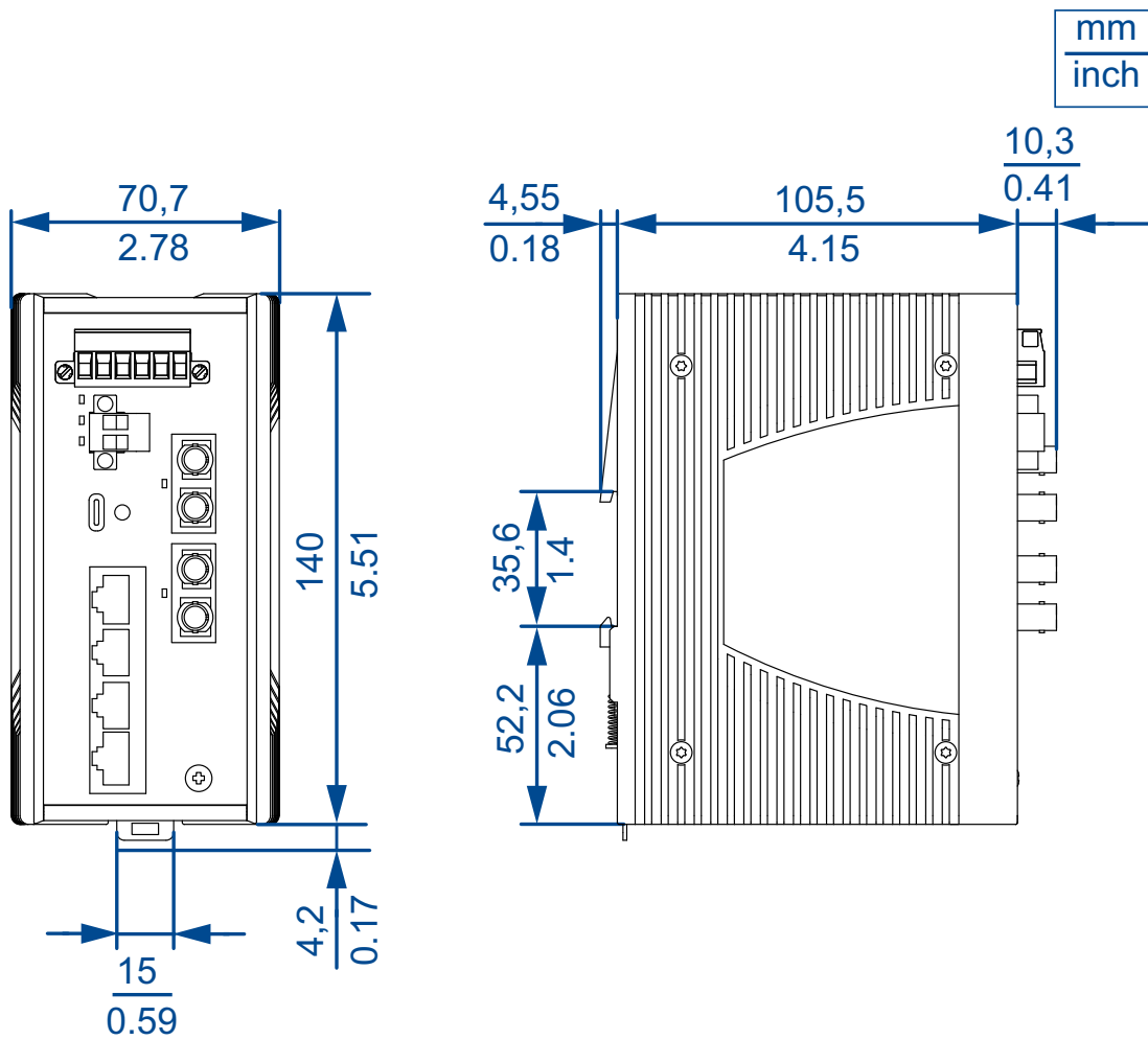
Abb. 27: Gerätevarianten im schmalen Metallgehäuse
