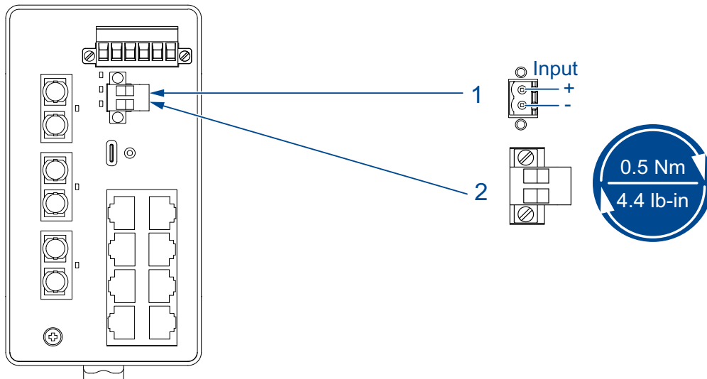
Abb. 19: (1) Anschluss am Gerät, (2) Klemmblock montiert am Gerät (Vorderansicht), Anzugsdrehmoment.
