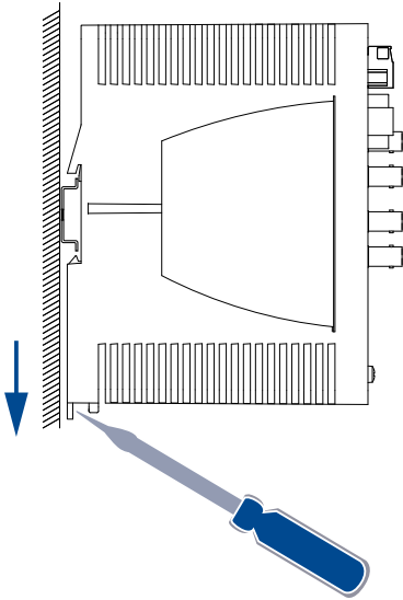
Abb. 23: Demontage von der Hutschiene
