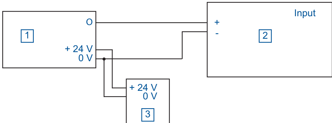
Abb. 20: Anschluss eines Sensors (3-Pol) mit gesonderter Spannungsversorgung 1 - Sensor 2 - BRS20/22/30/32/40/42/50/52 3 - Gesonderte Spannungsversorgung für Sensor
