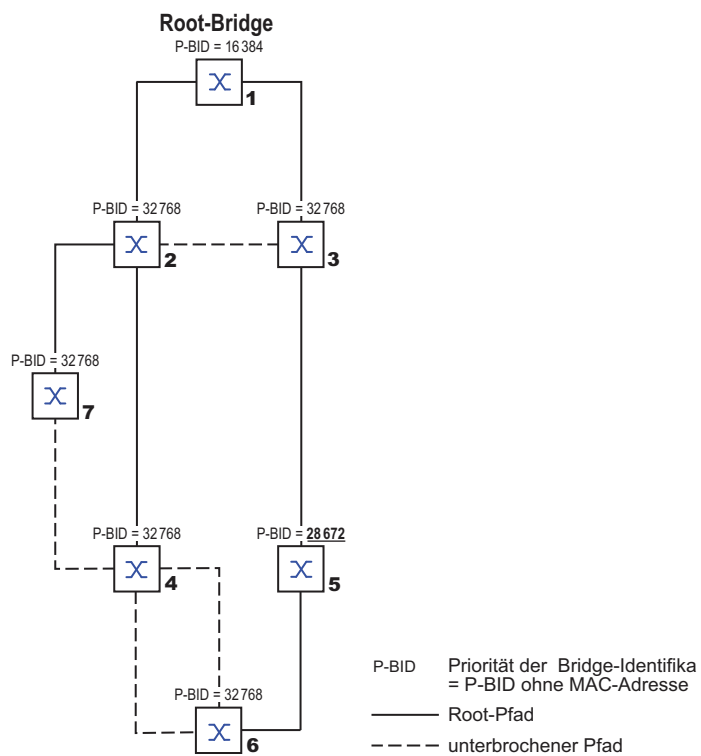
Abb. 39: Beispiel für die Manipulation des Root-Pfads
