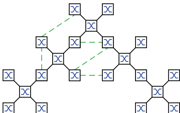
Abb. 27: Maschen-Topologie: Baum-Topologie mit physikalischen Schleifen
