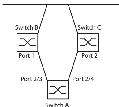
Abb. 43: Link-Backup Beispiel-Netzwerk
