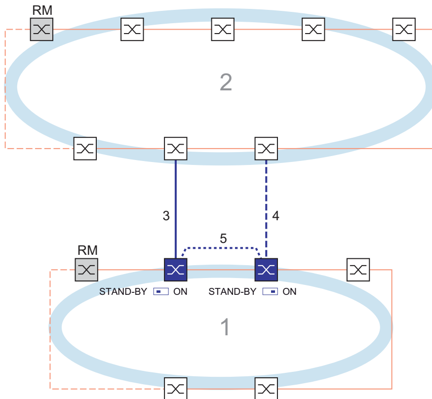
Abb. 50: Beispiel für die 2-Switch-Kopplung mit Steuerleitung
