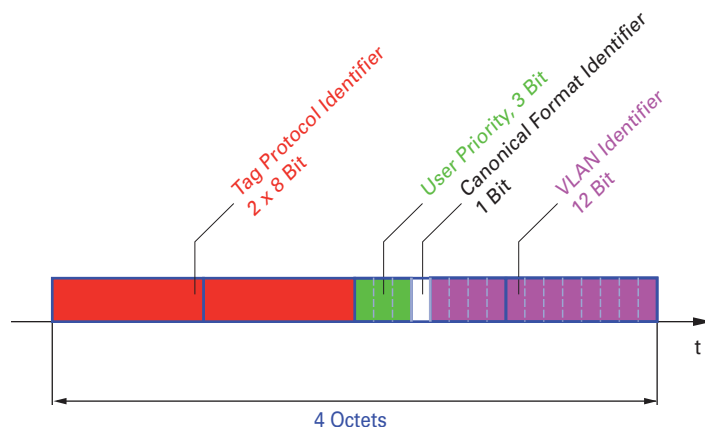
Abb. 22: Aufbau des VLAN-Tag
