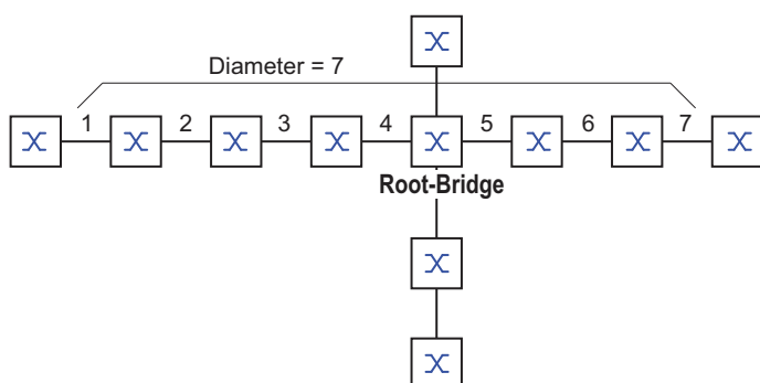
Abb. 35: Definition „Diameter“
