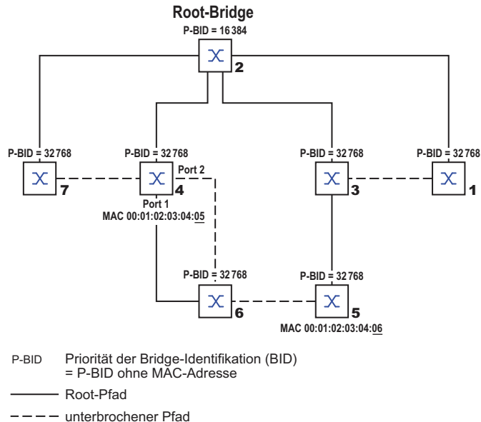
Abb. 40: Beispiel für die Manipulation der Baumstruktur
