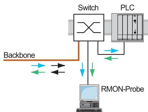
Abb. 54: Beispiel
