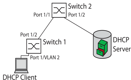
Abb. 55: Beispiel: DHCP-Schicht-2-Netz
