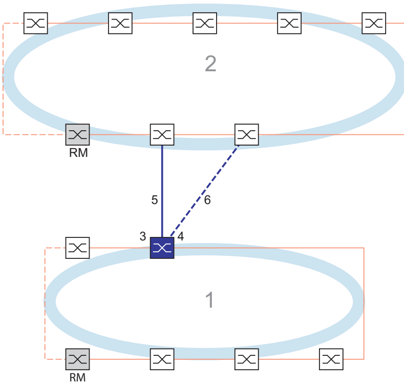
Abb. 44: Beispiel für die 1-Switch-Kopplung
