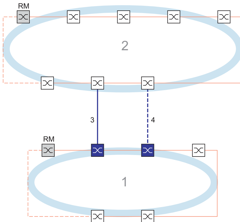
Abb. 46: Beispiel für die 2-Switch-Kopplung
