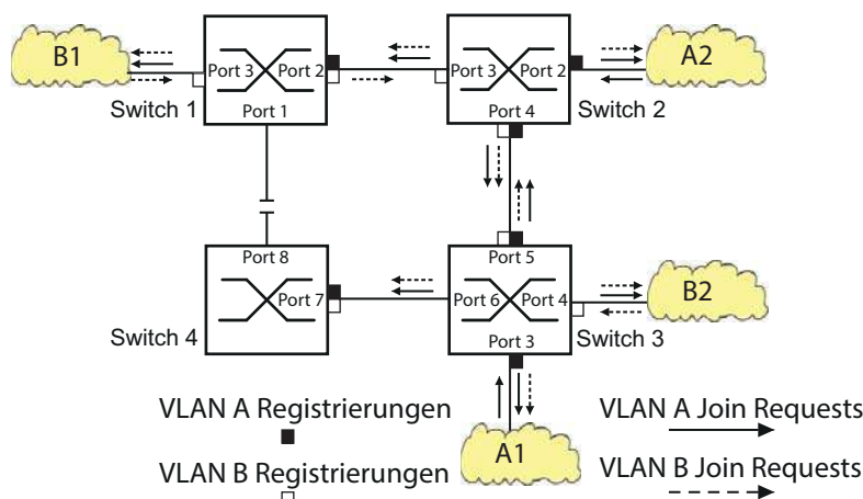
Abb. 57: MVRP -Beispiel-Netz für VLAN-Registrierung
