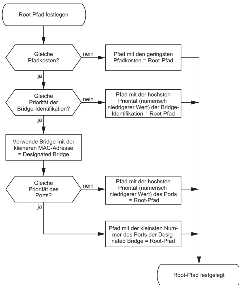
Abb. 37: Flussdiagramm Root-Pfad festlegen
