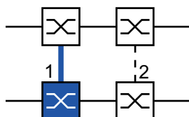
Abb. 47: 2-Switch-Kopplung, primäres Gerät
