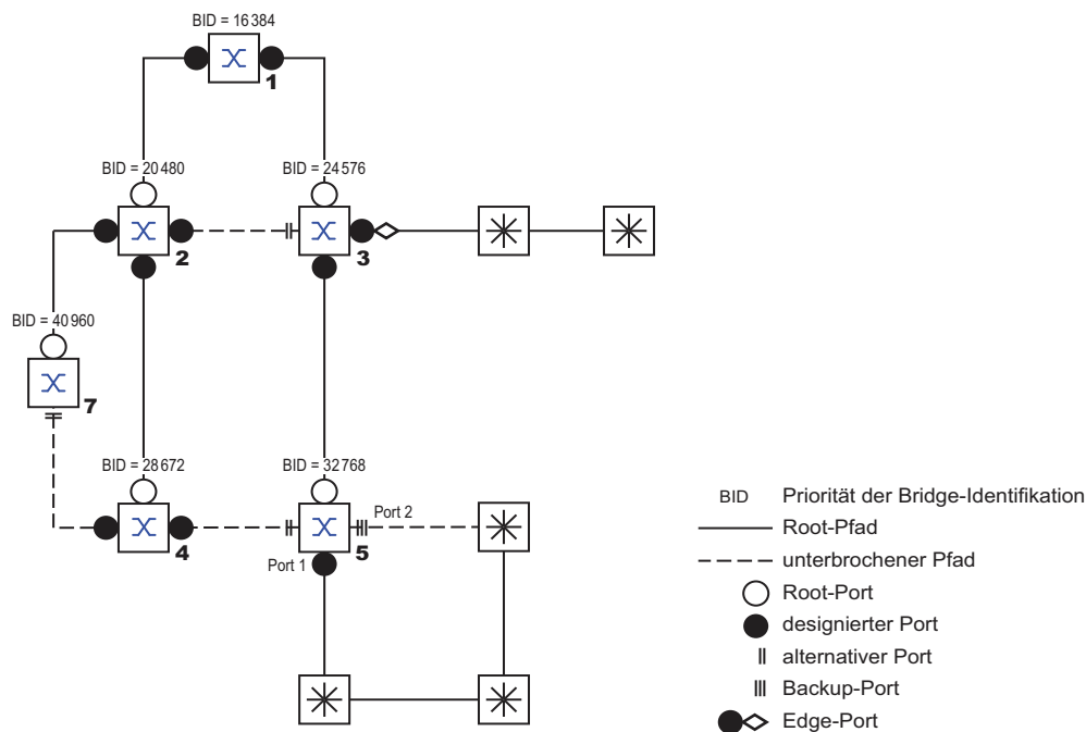
Abb. 41: Port-Rollen-Zuweisung
