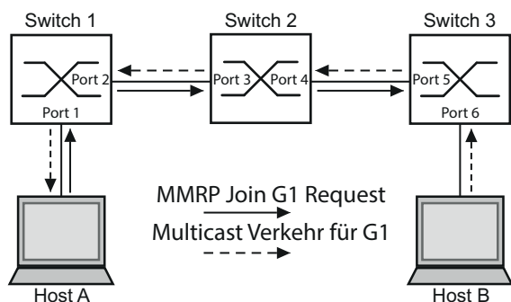
Abb. 56: MMRP -Netz für MAC-Adressen-Registrierung
