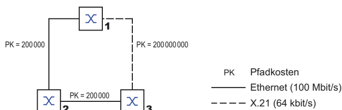
Abb. 33: Pfadkosten
