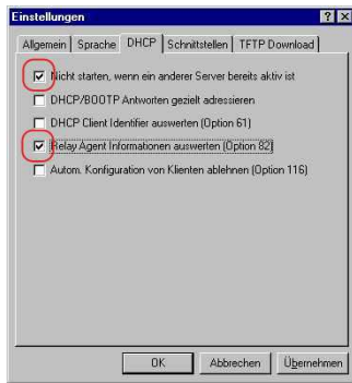
Abb. 69: DHCP-Einstellung
