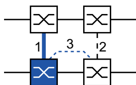
Abb. 51: 2-Switch-Kopplung mit Steuerleitung, primäres Gerät
