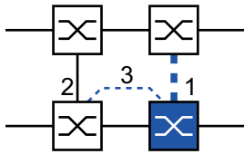
Abb. 52: 2-Switch-Kopplung mit Steuerleitung, Standby-Gerät
