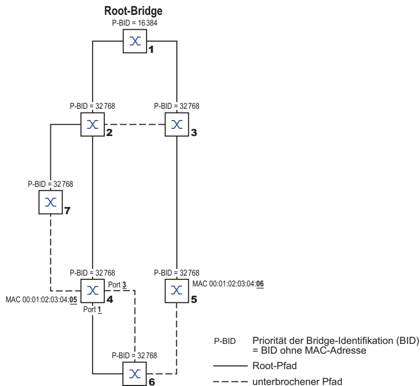
Abb. 38: Beispiel für die Bestimmung des Root-Pfads
