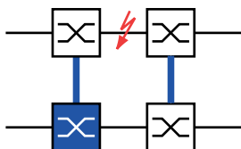
Abb. 53: Erweiterte Redundanz
