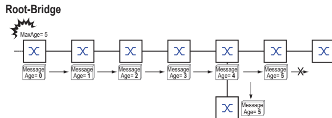
Abb. 36: Übertragung einer STP-BPDU in Abhängigkeit von MaxAge
